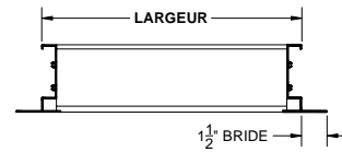
MODÈLE 2455 CADRE: EN "L" À BRIDE (FM)
